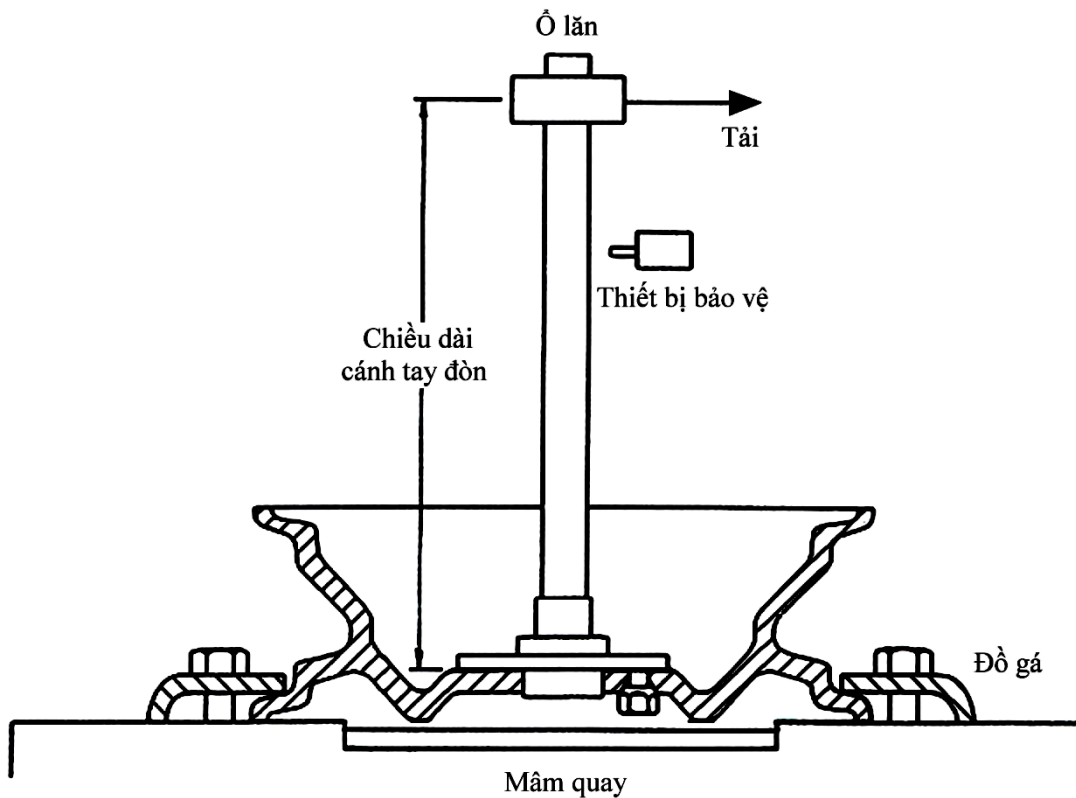
Hình B.1 : Thiết bị thử mài góc điển hình
