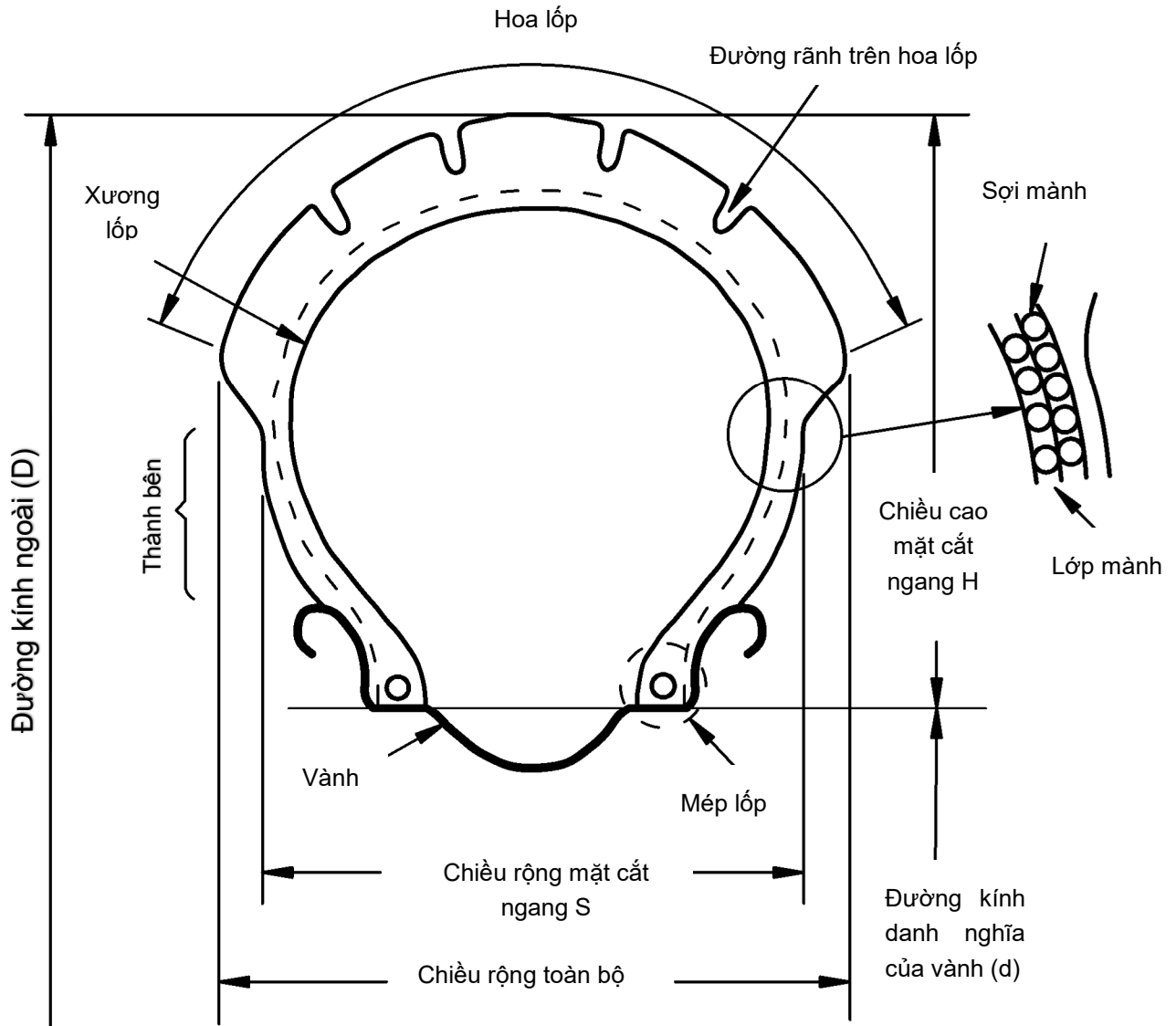
Hình 1. Mặt cắt ngang của lốp
