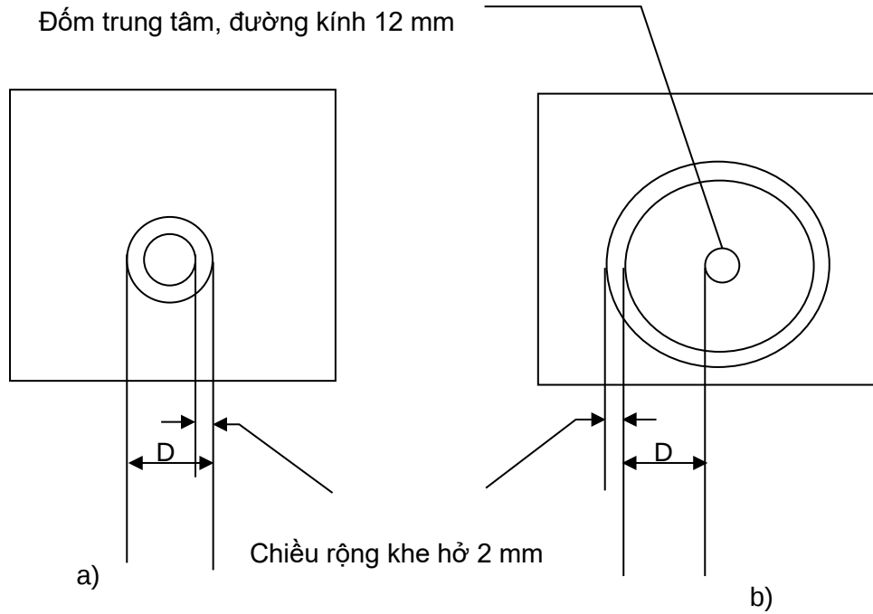
Hình 13 - Các kích thước của bia
