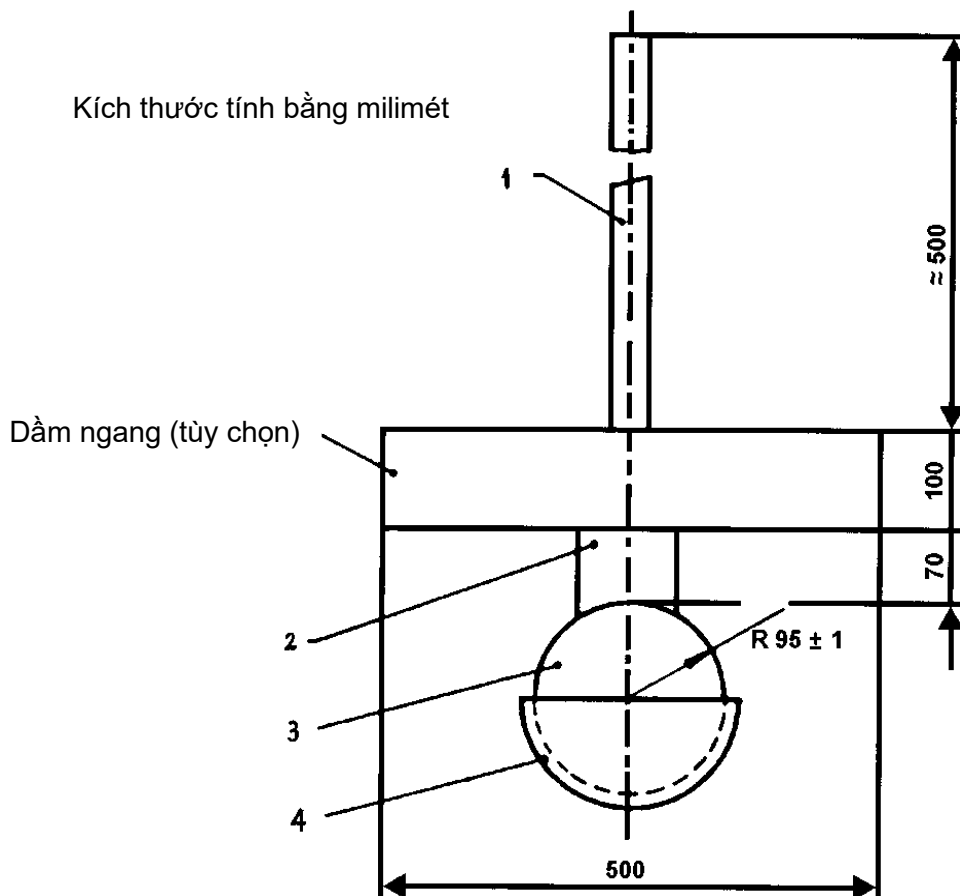
Hình 2. Chùy thử
