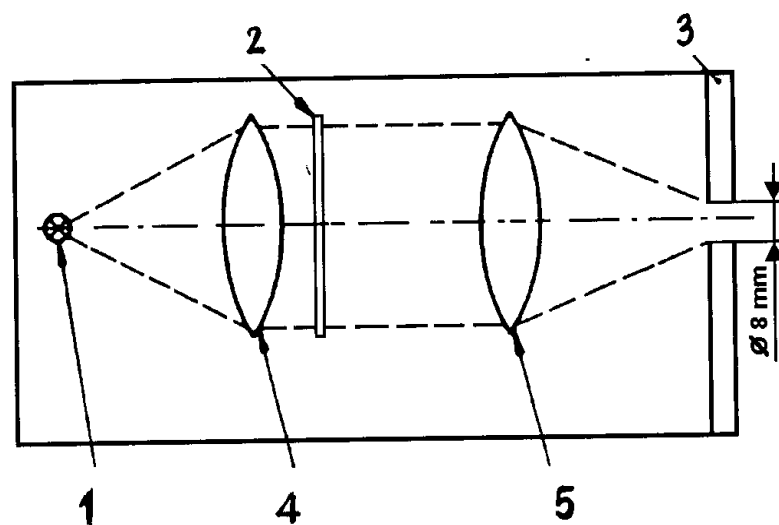
Hình 8 - Sơ đồ biểu diễn độ méo quang
