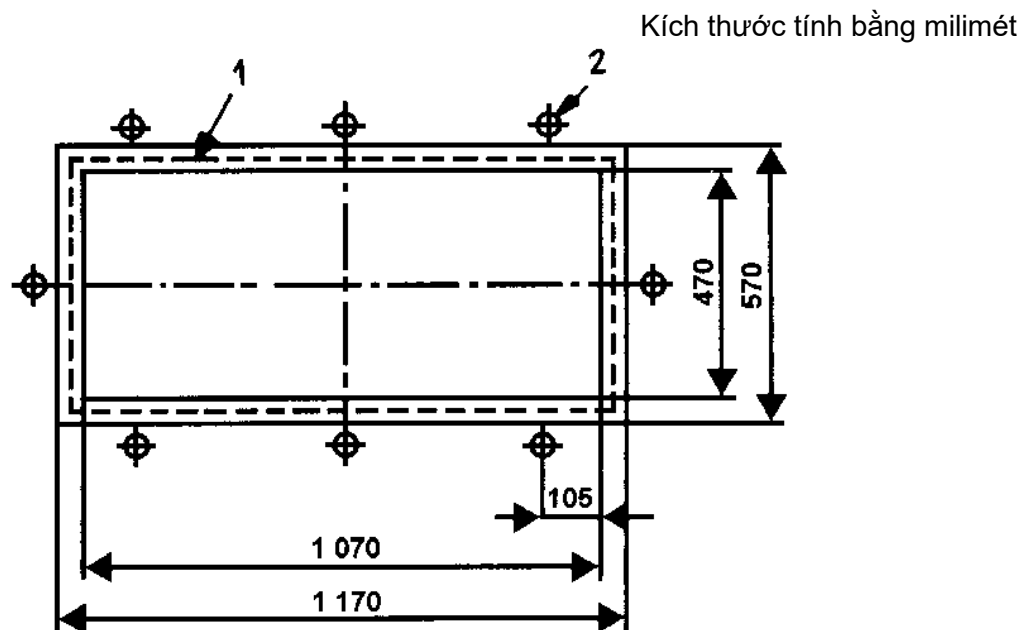
Hình 3 - Giá đỡ thử bằng chùy thử
