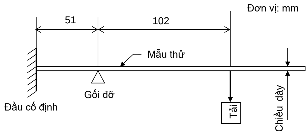
Hình 23 : Phương pháp gá đặt mẫu thử
