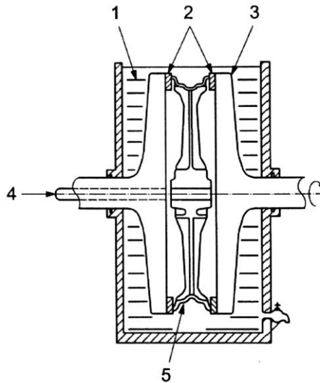
Hình G.1 - Thiết bị thử độ kín khít đối với vành lắp lớp không sẫm
